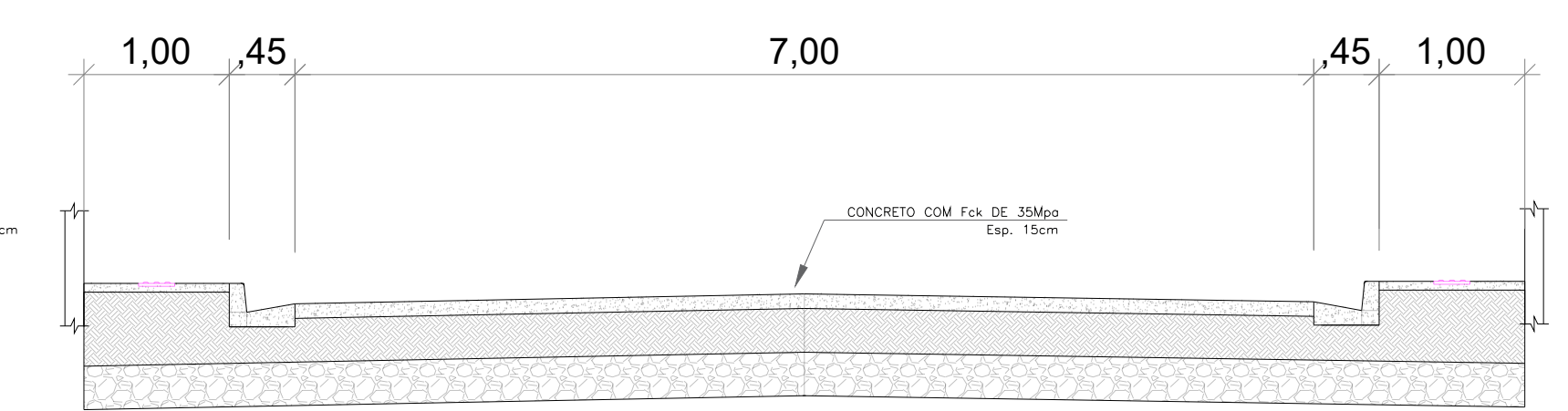
Det. Corte - Calçada Esc.: 1/20
