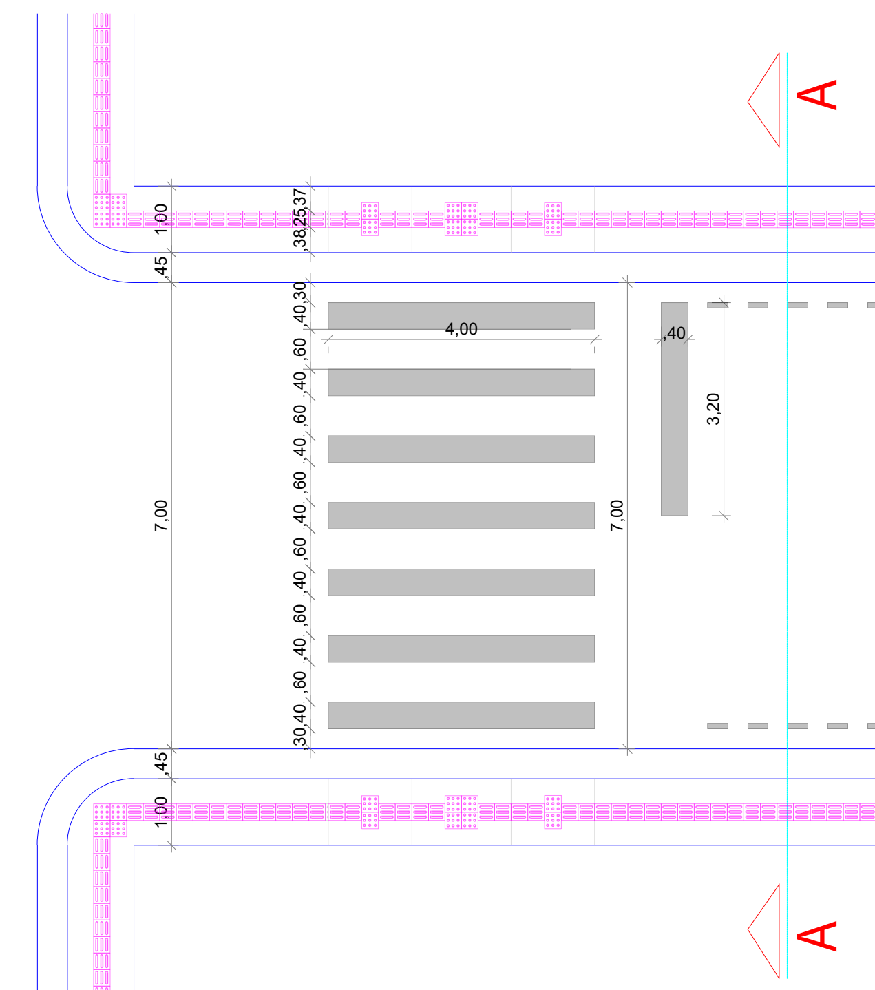
DETALHES SINALIZAÇÃO HORIZONTAL Esc.: 1/100
