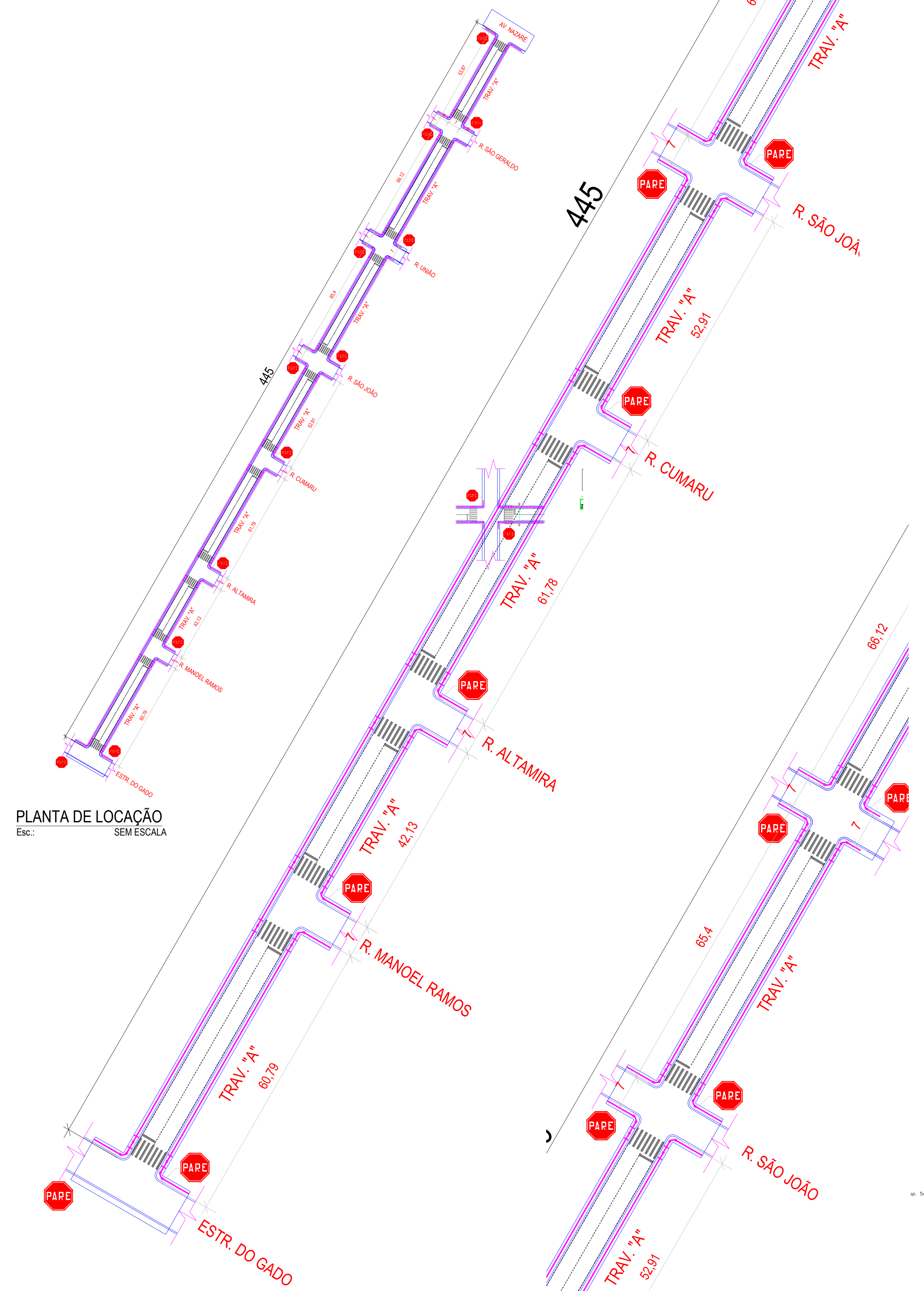
PLANTA BAIXA - TRECHO 01 - ENTRE ESTR. DO GADO E RUA SÃO JOÃO Esc.: 1/500
