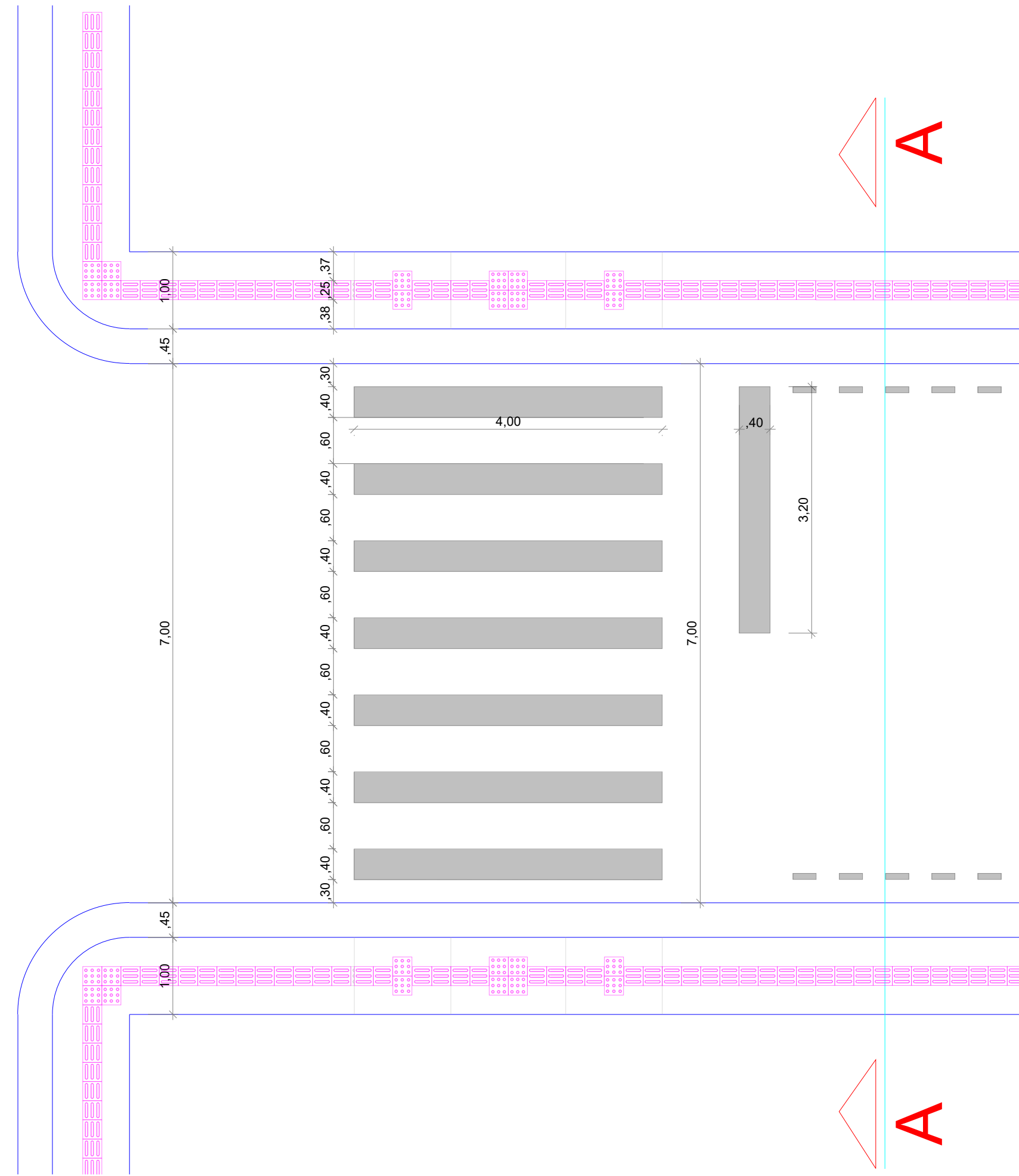
DETALHES SINALIZAÇÃO HORIZONTAL Esc.: 1/100
