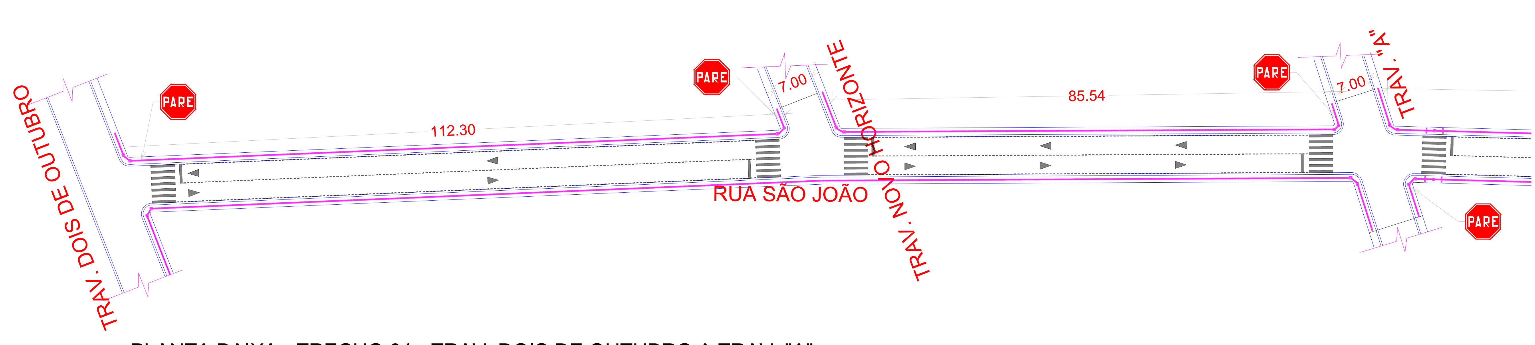
PLANTA BAIXA - TRECHO 01 - TRAV. DOIS DE OUTUBRO A TRAV. "A" Esc.: 1/500
