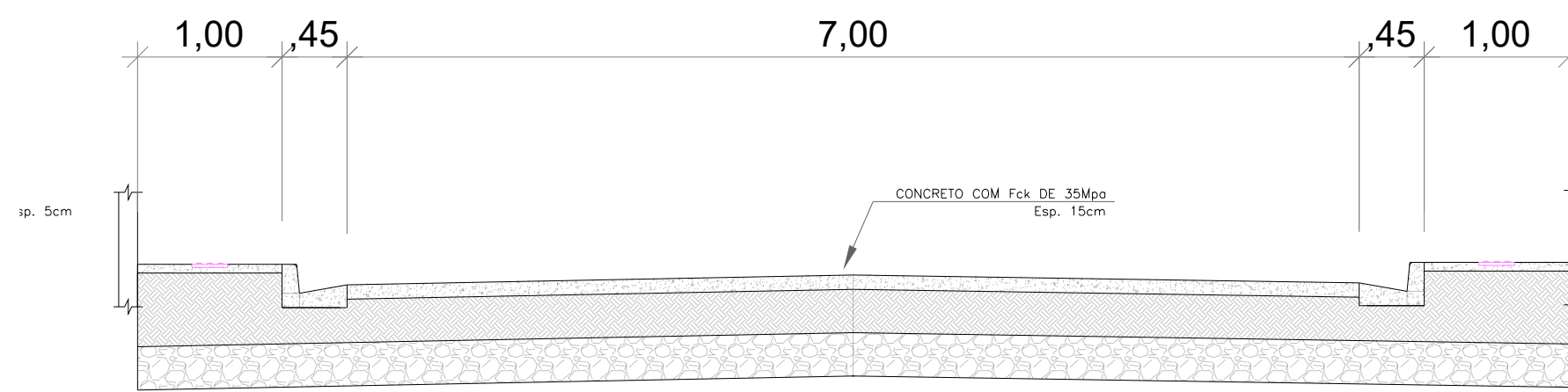
Det. Corte - Calçada Esc.: 1/20
