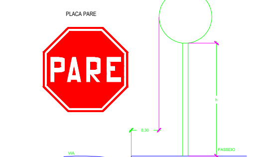
DETALHES SINALIZAÇÃO VERTICAL Esc.: 1/100
